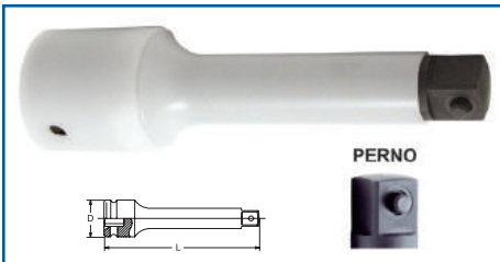
PROLUNGA CON RIVESTIMENTO
