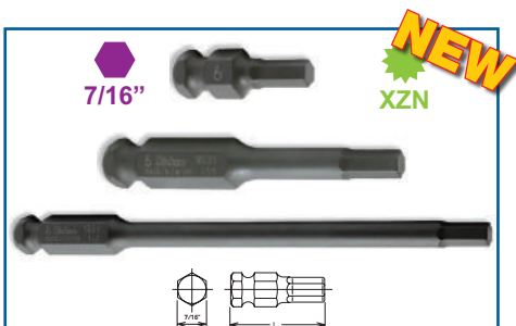
INSERTO CON MASCHIO XZN
