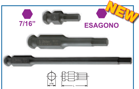
INSERTO CON MASCHIO ESAGONALE
