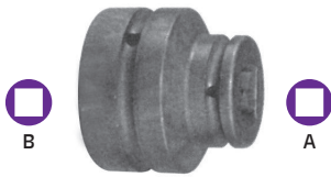
RIDUZIONI PER BUSSOLE "POWER IMPACT" FEMMINA/FEMMINA
