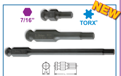
INSERTO CON MASCHIO TORX®
